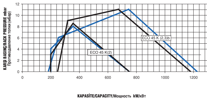
ECO45 K ÇALIŞMA DİYAGRAMI/WORKING DIAGRAM Диаграмма производительности
